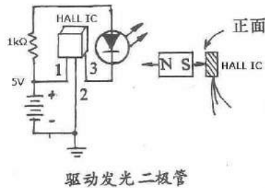
驱动发光二极管
