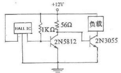
驱动 4A 直流负载
