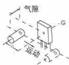
②平动工作方式
